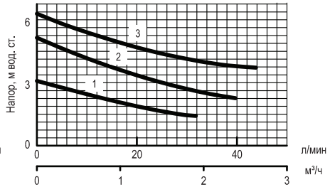
Диаграммы характеристик насосов АСР 25-60тип2, АСР 32-60тип2
