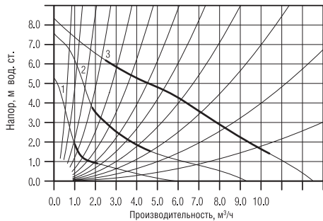
Диаграммы характеристик насоса АСР 32-80тип2
