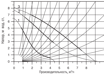
Диаграммы характеристик насоса АСР 25-80тип2
