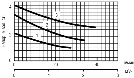
Диаграммы характеристик насосов АСР 25-40тип2, АСР 32-40тип2
