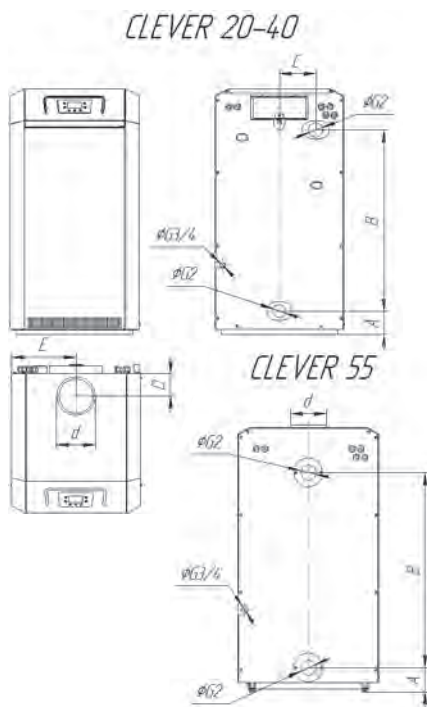
Рис.3. Присоединительные размеры
